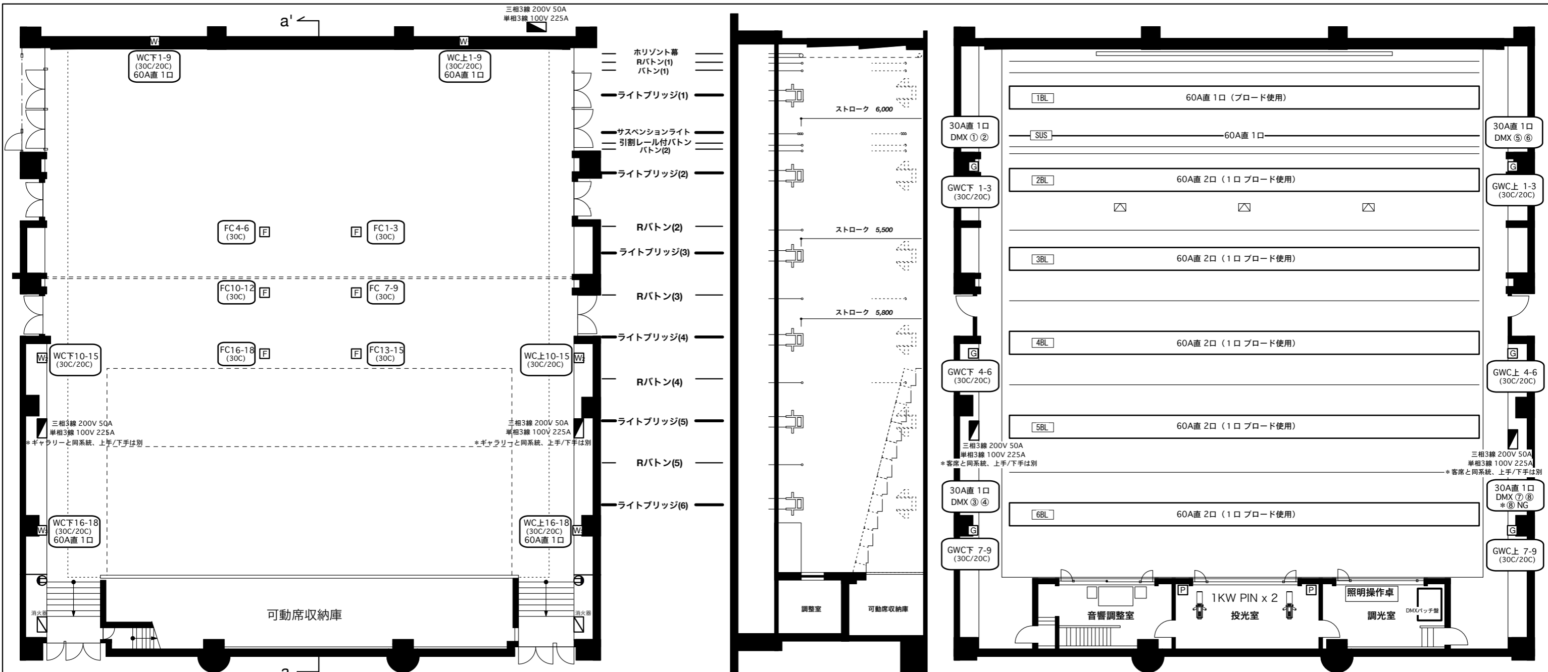
1階 平面図
